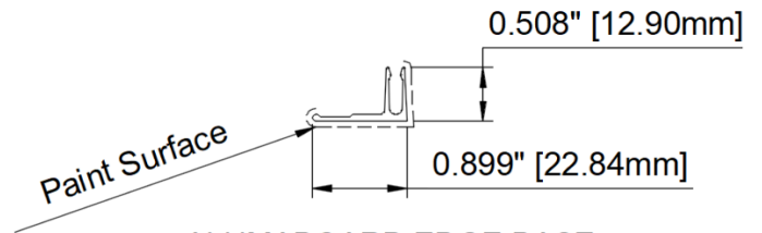
ALUMABOARD EDGE BASE
