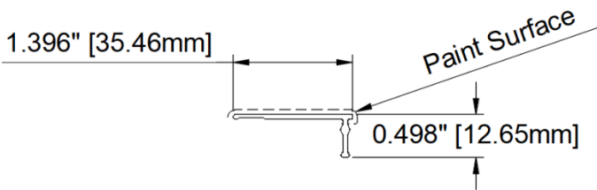
ALUMABOARD EDGE TOP
