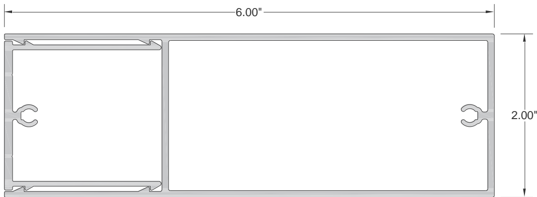
2" X 6" Batten
