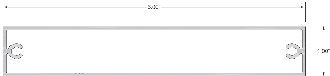
1" x 6" Batten
