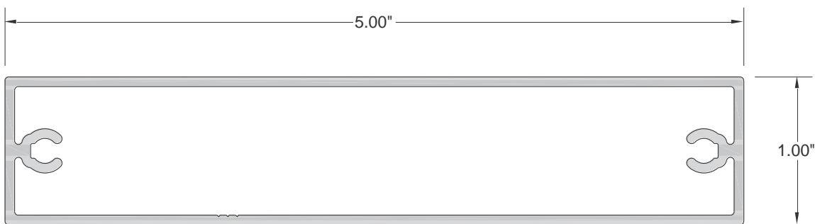
1" x 5" Batten
