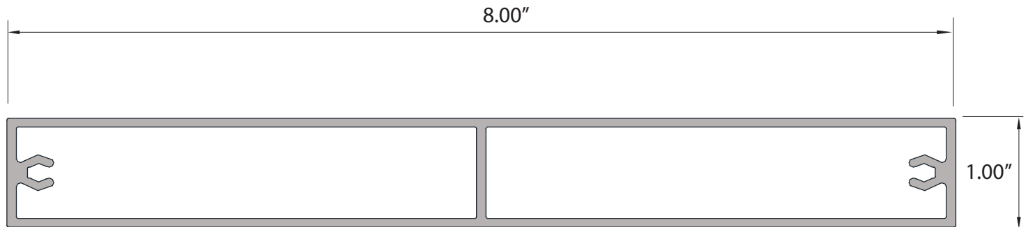
1" x 8" Batten
