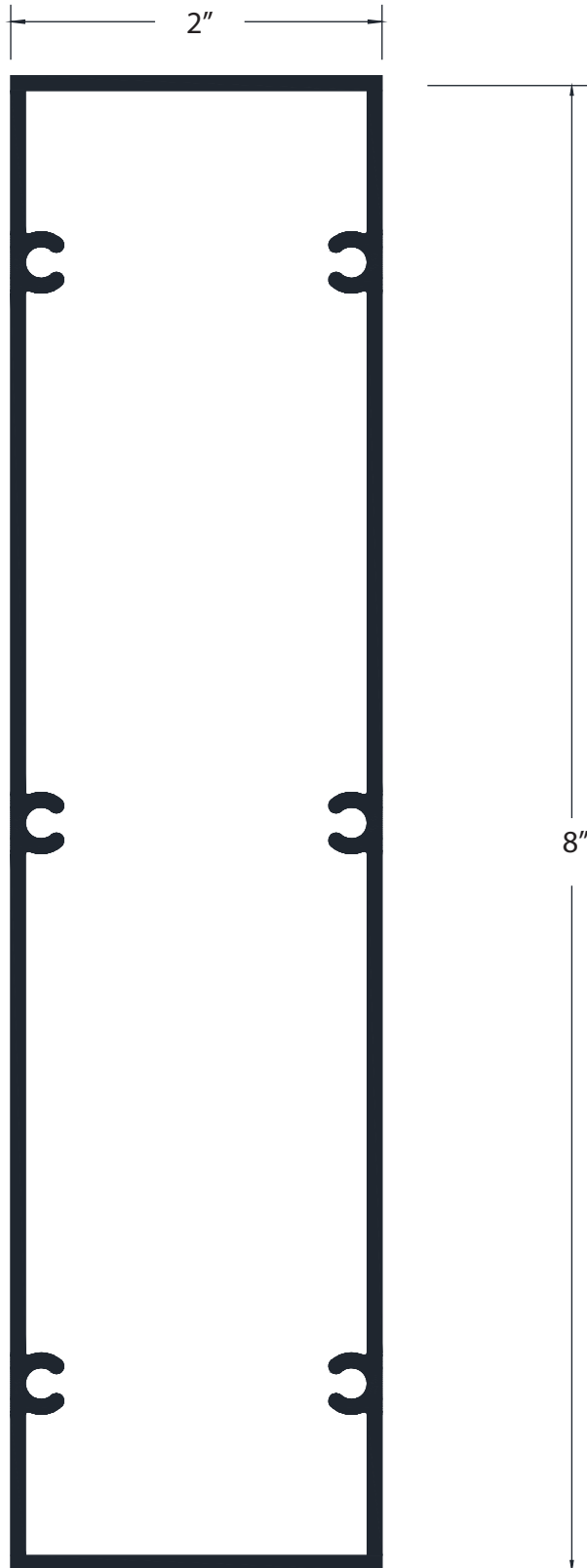
2"x 8" Batten
