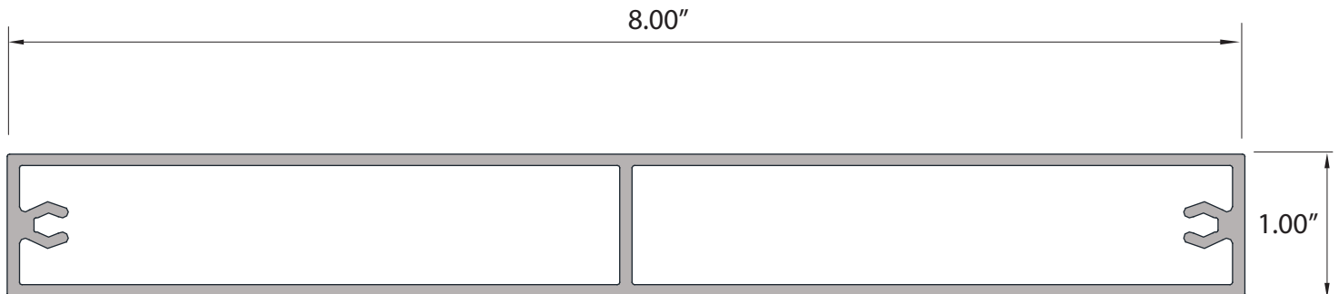
1" x 8" Batten
