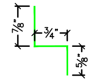
ZEE SPACER
